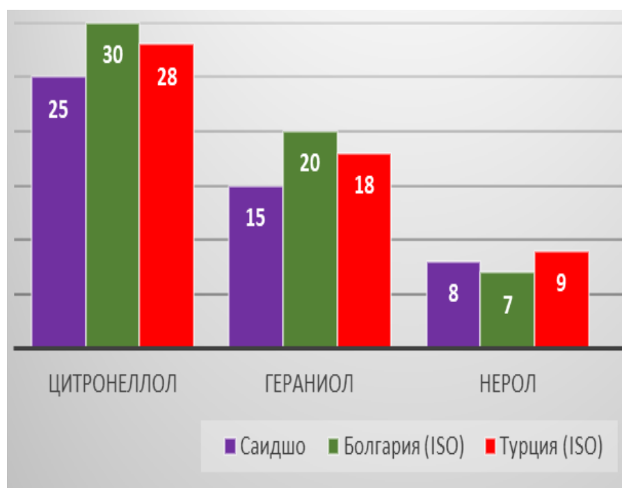
Рисунок 4.4. Сравнительный анализ компонентного состава эфирного масла R. damasena М. и эталонных образцов Болгарии и Турции (по данным стандарта ISO)
