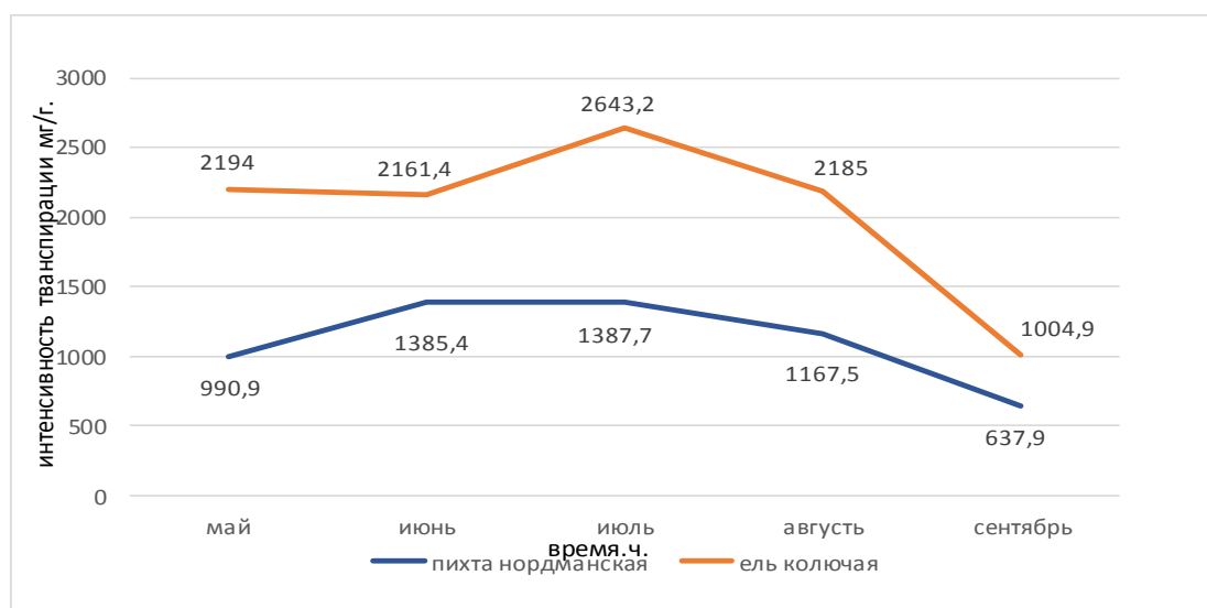
Рисунок 1. Интенсивность транспирации у Пихты нордманской и Ели колючей с мая по сентябрь (2022 г.)
