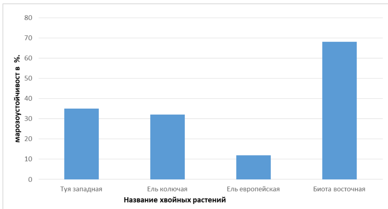
Рисунок 4.2.1. - Морозоустойчивость хвойных растений в условиях Западного Памира
