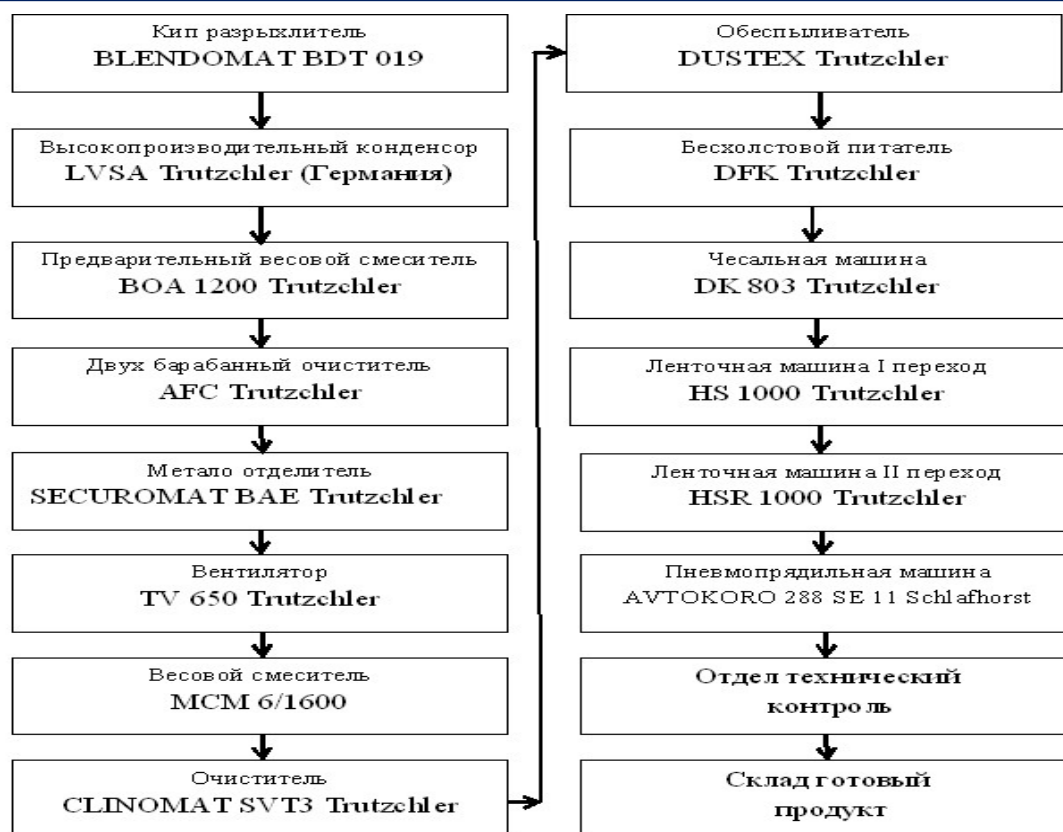
Рисунок 5 – Схема технологического процесса выработки пряжи пневмомеханическим способом на ОАО Ресандаи Кулоб
