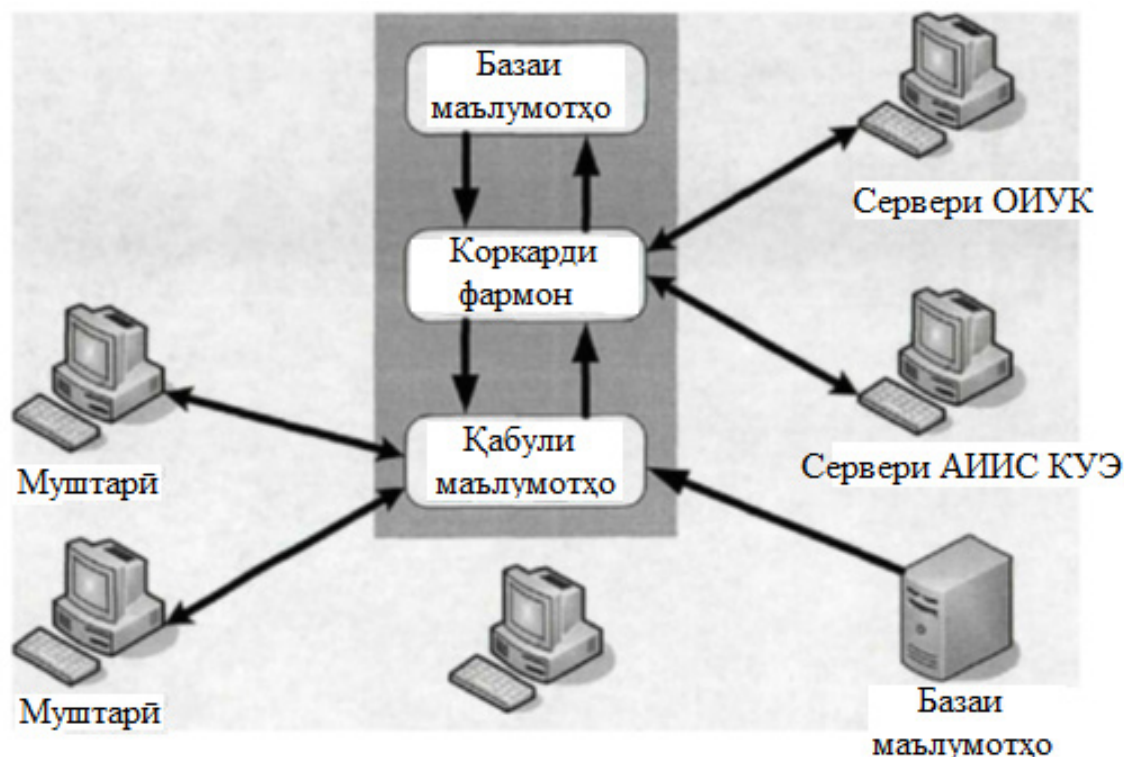
Расми 2. Нақшаи таъмини техникии низоми мониторинги талафоти нерӯи барқ.
